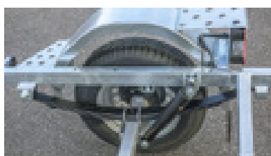
AKU BX750 -mallissa on 4-lehtiset jouset. Valorunko toimii askelmana.
